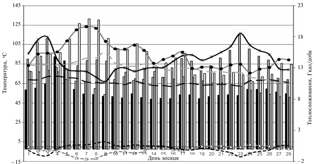
Рис. 5. Порівняння параметрів теплопостачання навчального корпусу технічного університету (НТУУ “КПІ”) за лютий у 2009 і 2010 рр.: ■ — фактичне теплоспоживання за лютий 2009 р.; ▨ — фактичне теплоспоживання за лютий 2010 р.; — — фактична температура подачі теплоносія протягом лютого 2009 р.; - - - фактична температура подачі теплоносія протягом лютого 2010 р.; - - - - температура навколишнього середовища за лютий 2009р.; - -△- - температура навколишнього середовища за лютий 2010 р.; * — необхідна температура подачі теплоносія протягом лютого 2009 р.; ● — необхідна температура подачі теплоносія протягом лютого 2010 р.; ▨ — необхідне теплоспоживання за лютий 2009 р.; ■ — необхідне теплоспоживання за лютий 2010 р.
