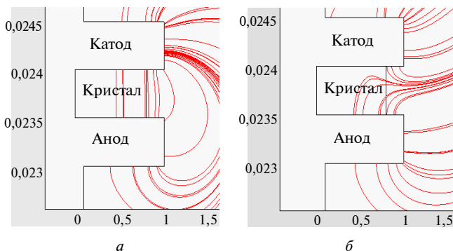
Рис. 1. Картина електричного поля в конструкції стабілітрона Д818Д зі скляним корпусом; потенціал на верхньому екрануючому електроді: a – 9 В; b – 10 кВ
